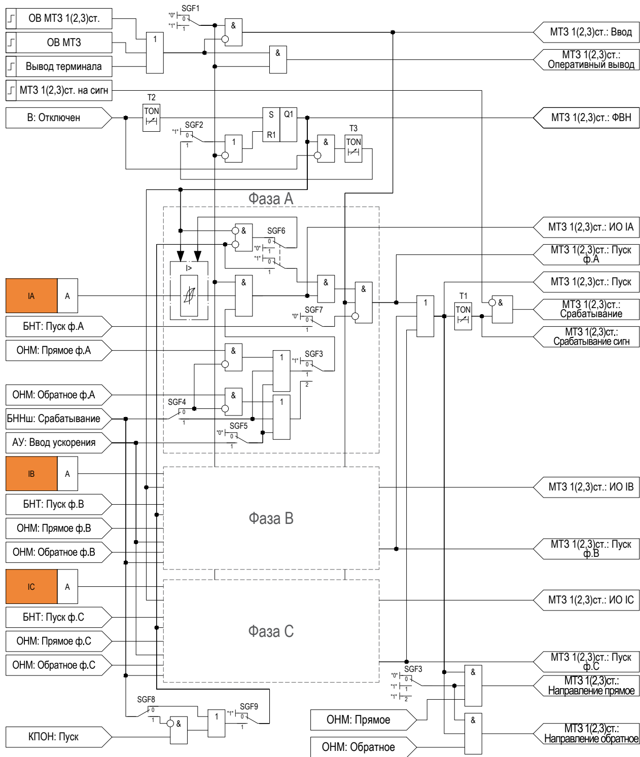
Рисунок 2.15 – Функциональная схема ступеней «MT3 1 ст», «MT3 2 ст», «MT3 3 ст»
